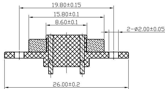
SEC A-A
