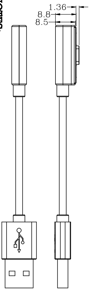
PVC圆线(φ3.0)四芯
