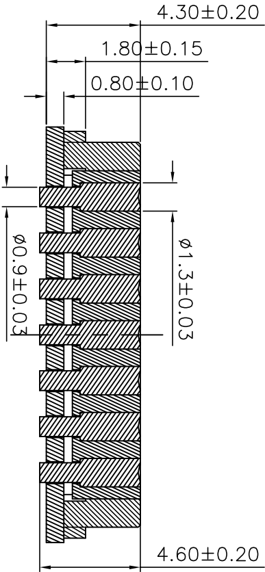
截面 AA-AA
