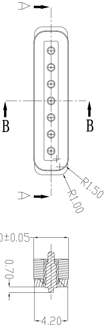
截面 B-B
