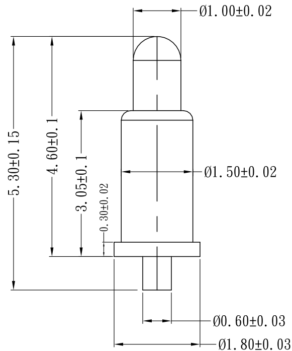
工作高度 working. stroke
