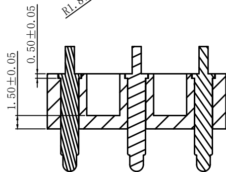
截面A-A
